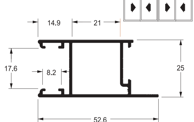
SU-039 0,488 kg/m
