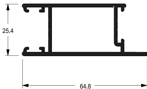
SU-245 0,638 kg/m
