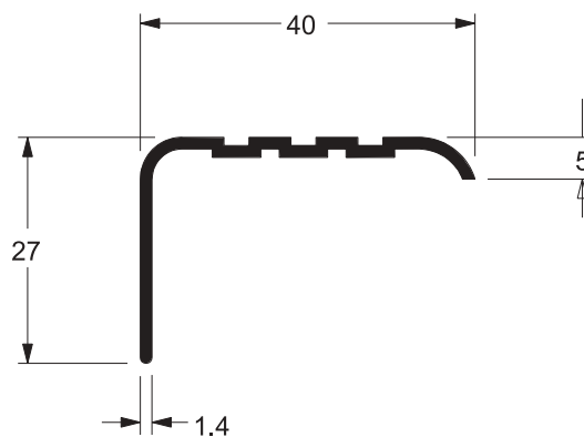
ME-013 0,267 kg/m
