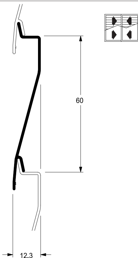
Veneziana ventilada
