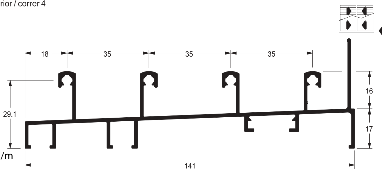
Marco inferior / correr 4
