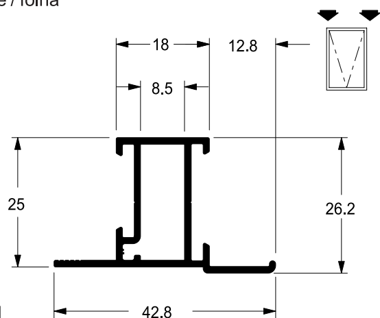
Montante / folha
