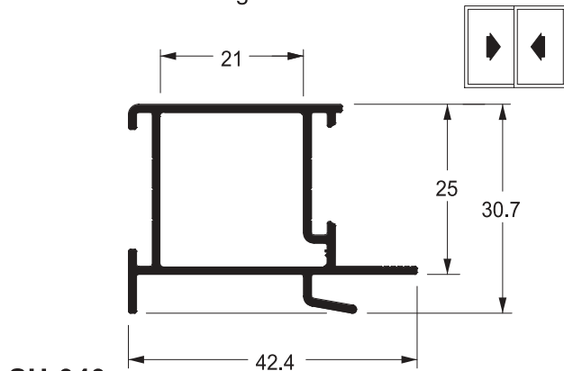
SU-040 0,429 kg/m
