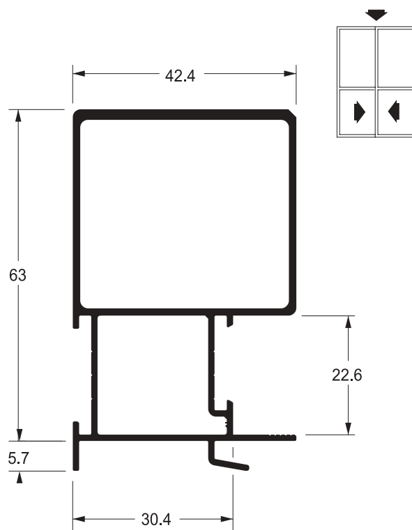
SU-047 0,958 kg/m
