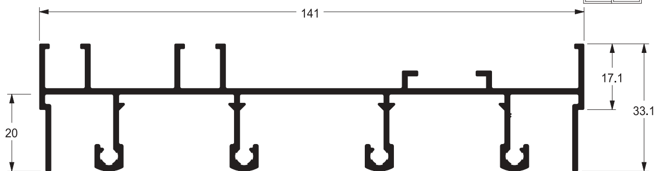
Marco superior / correr 4
