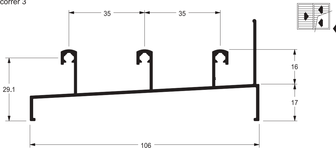
Marco inferior / correr 3
