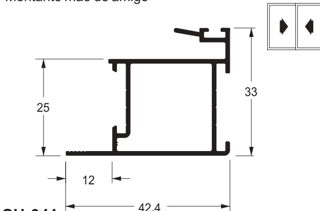
SU-041 0,466 kg/m
