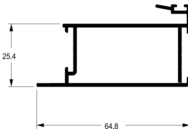
SU-242 0,699 kg/m
