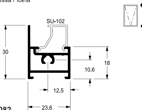
Travessa / folha
