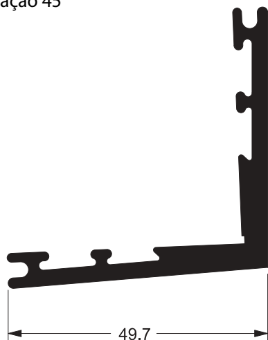
Cantoneira Ligação 45°
