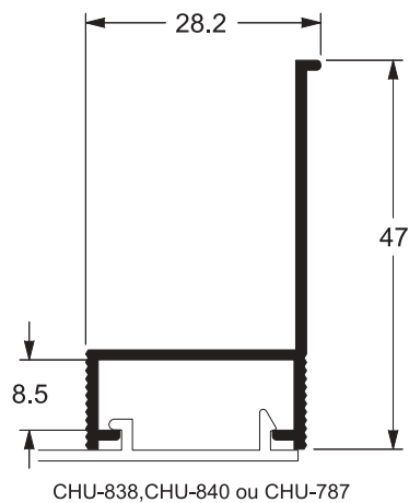
CM-151 0,244 kg/m
