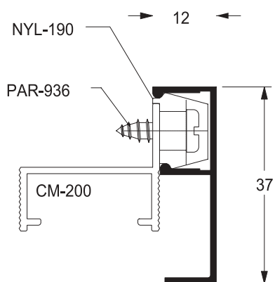
MP-347 0,202 kg/m
