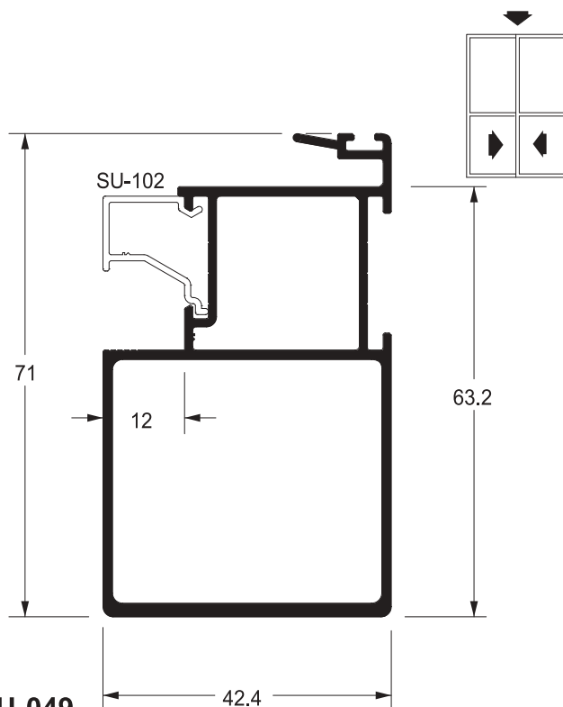
SU-049 0,866 kg/m
