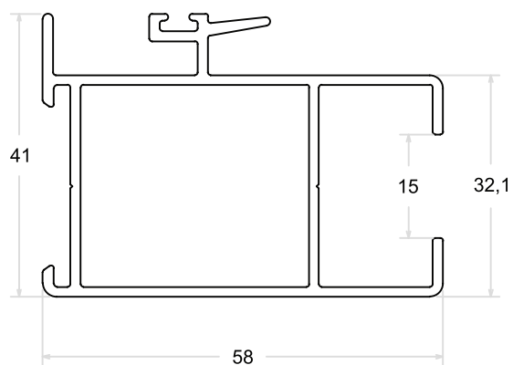
LG - 128 | PESO: 0,900 Kg/m Folha Mão de Amigo - Sem Baguete
