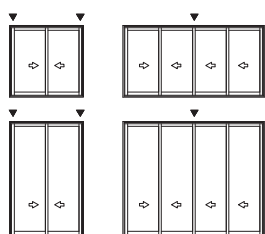
LG - 132 | PESO: 0,799 Kg/m Folha Lateral Vertical - Sem Baguete
