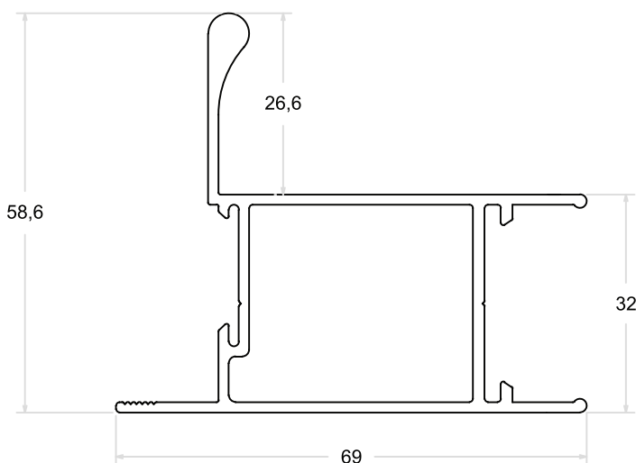
LG - 017 | PESO: 1,005 Kg/m
