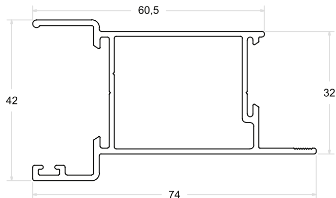
LG - 051 | PESO: 0,830 Kg/m
