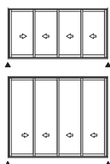
LG - 072 PESO: 1,148 Kg/m Marco Lateral Vertical
