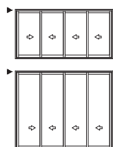
LG - 070 PESO: 2,088 Kg/m Marco Superior Horizontal
