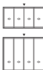
LG - 133 | PESO: 0,902 Kg/m Folha Central Vertical - Sem Baguete
