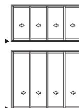
LG - 160 PESO: 1,906 Kg/m Marco Inferior Horizontal
