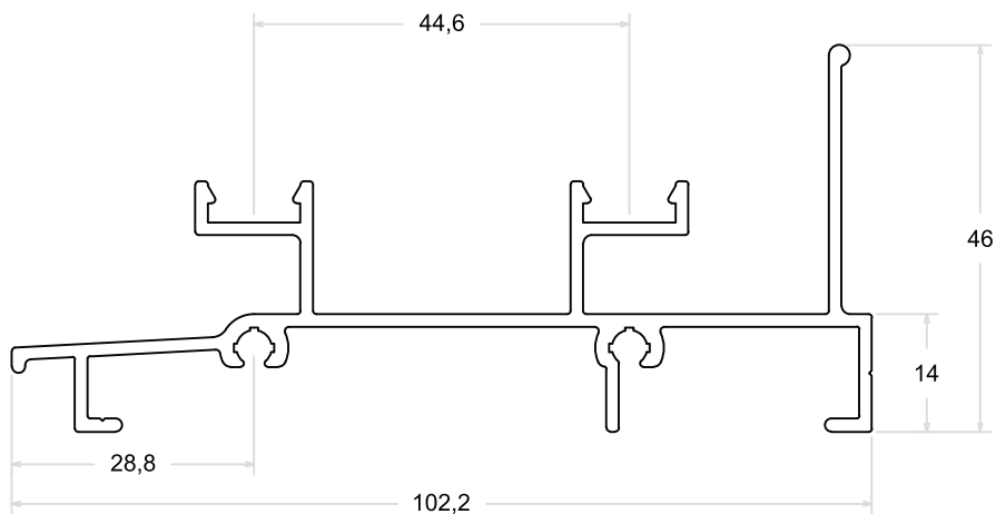
LG - 159 | PESO: 1,099 Kg/m
