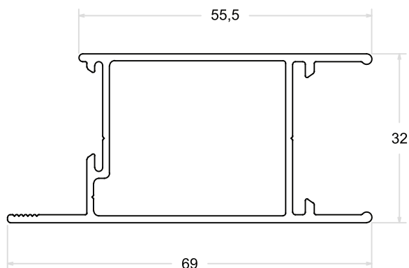
LG - 050 | PESO: 0,729 Kg/m
