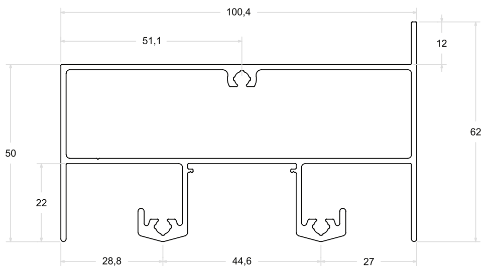
LG - 004 | PESO: 1,774 Kg/m
