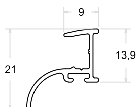
LG - 092 | PESO: 0,145 Kg/m
