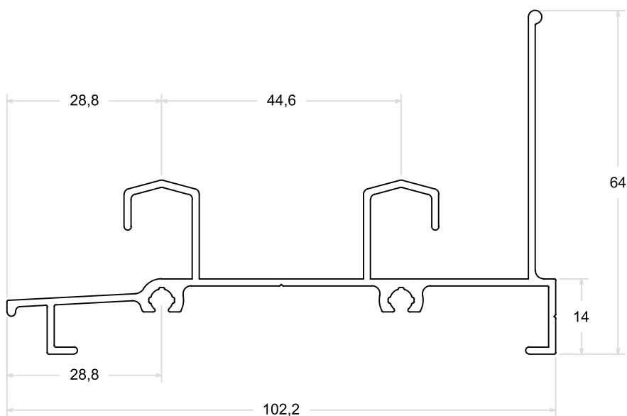
LG - 047 | PESO: 0,967 Kg/m
