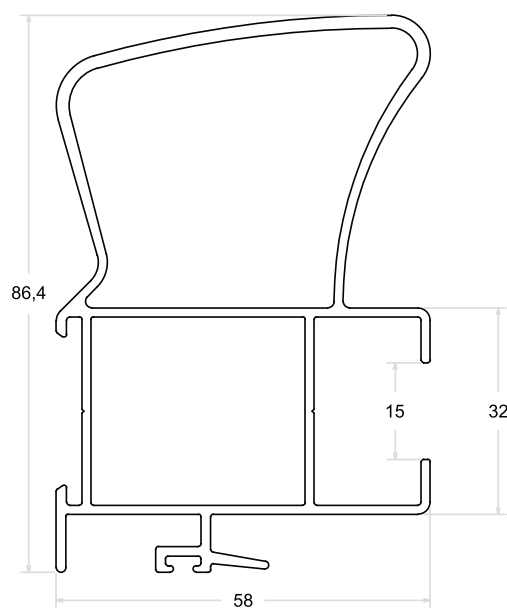
LG - 127 | PESO: 1,571 Kg/m Folha Mão de Amigo com Reforço - s/ Baguete
