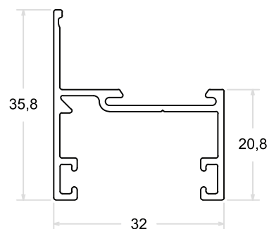
LG - 083 | PESO: 0,368 Kg/m
