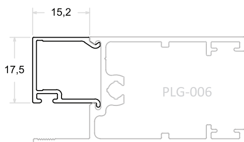
LG - 059 | PESO: 0,157 Kg/m
