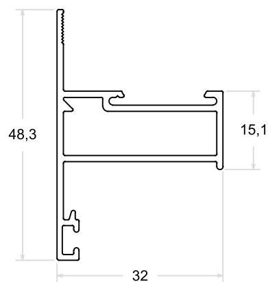
LG - 085 | PESO: 0,452 Kg/m
