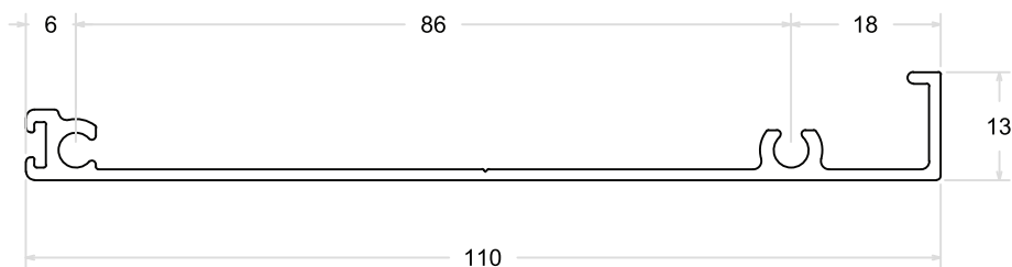
LG - 200 | PESO: 0,570 Kg/m Travessa Intermediária - Integrada
