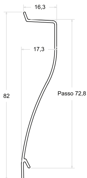
VZ - 082 | PESO: 0,280 Kg/m
