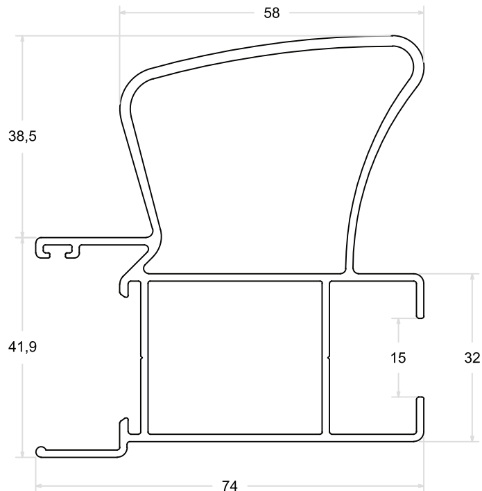
LG - 136 | PESO: 1,601 Kg/m
