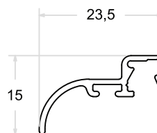
LG - 091 | PESO: 0,135 Kg/m
