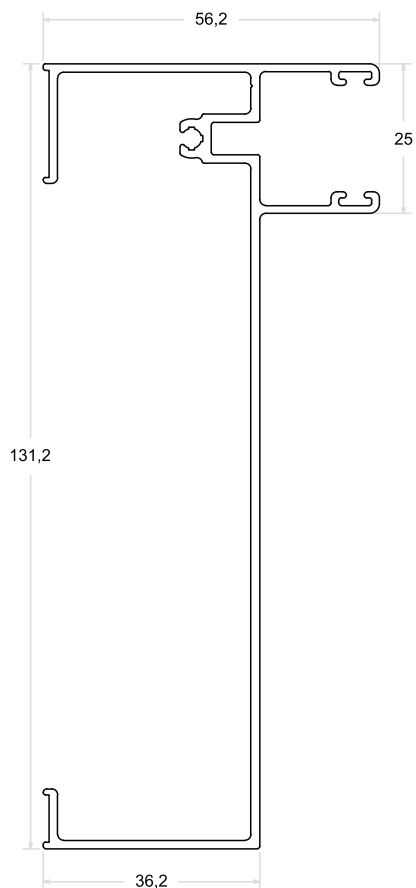
LG - 236 | PESO: 1,185 Kg/m
