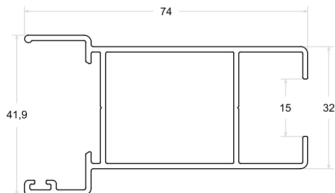
LG - 133 | PESO: 0,902 Kg/m Folha Central Vertical - Sem Baguete
