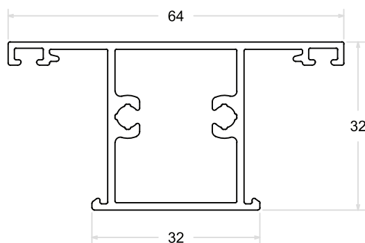
LG - 074 | PESO: 0,761 Kg/m
