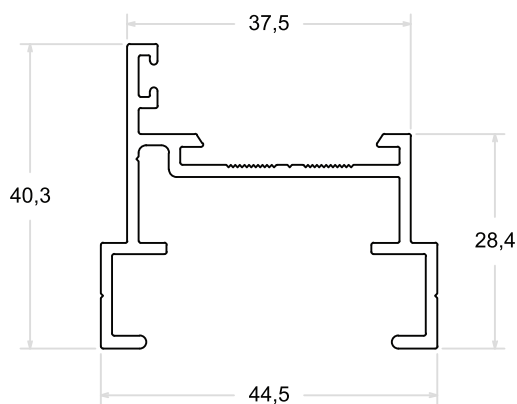
LG - 056 | PESO: 0,588 Kg/m
