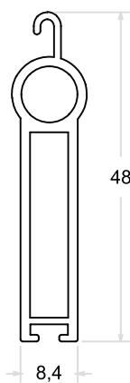
IT - 009 | PESO: 0,41 Kg/m
