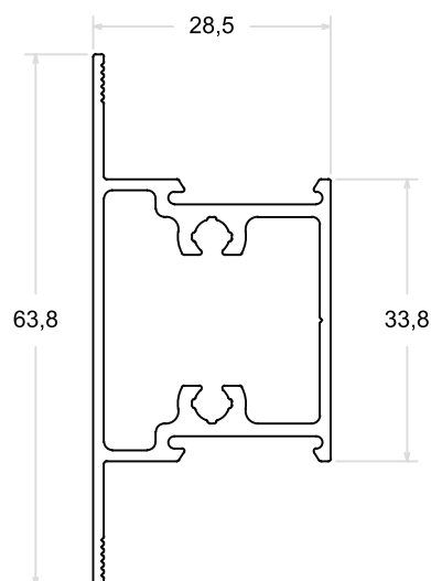
LG - 055 | PESO: 0,706 Kg/m
