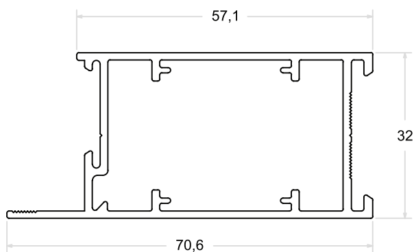
LG - 043 | PESO: 0,877 Kg/m
