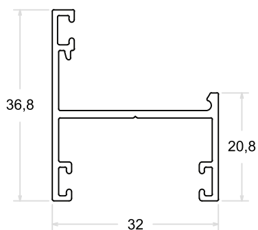
LG - 068 | PESO: 0,369 Kg/m
