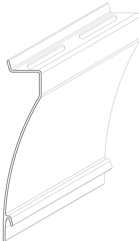
VZ - 106VT | PESO: 0,405 Kg/m
