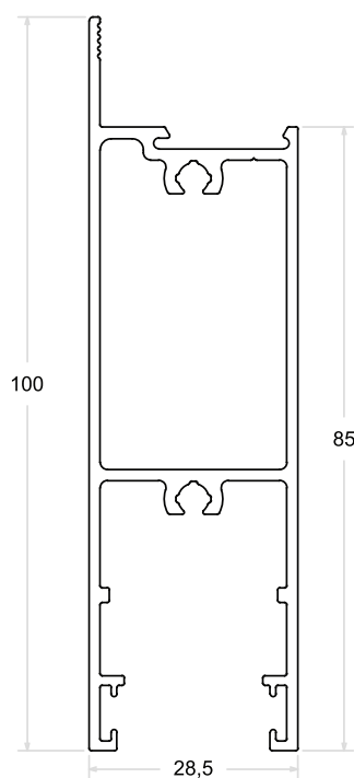
LG - 007 | PESO: 1,160 Kg/m
