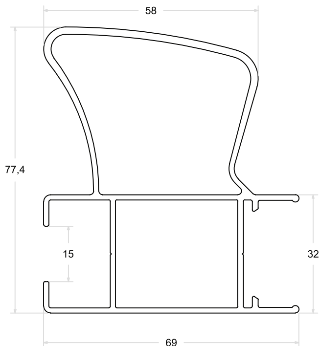
LG - 135 | PESO: 1,519 Kg/m
